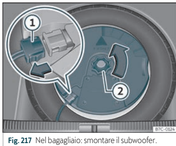
Fig. 217 Nel bagagliaio: smontare il subwoofer.
