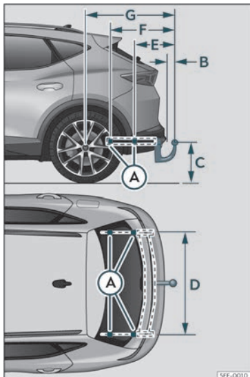
Fig. 186 Quote e punti di fissaggio per il montaggio successivo di un dispositivo di traino.
