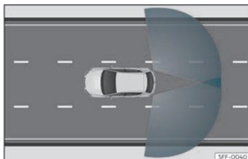
Fig. 149 Zone di rilevamento dei sensori
