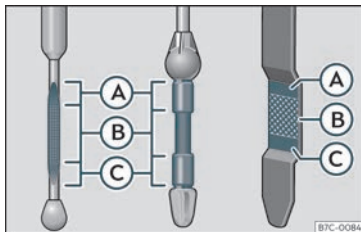
Fig. 203 Asta di misurazione livello olio motore.
