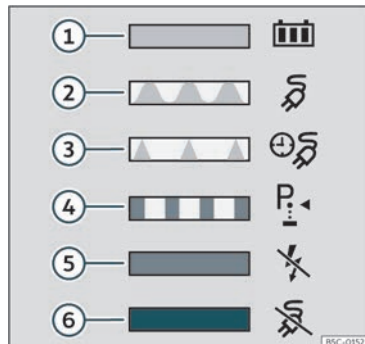
Fig. 191 All'interno del coperchio della presa di ricarica della batteria: adesivo con informazioni sull'indicatore del processo di ricarica.
