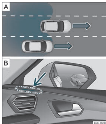
Fig. 168 Rappresentazione schematica: A ) Situazione in un sorpasso nella corsia centrale e spostamento successivo nella corsia di destra. B ) Indicazione dell'assistente al cambio corsia sulla spia di controllo di destra.
