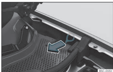
Fig. 192 Tra l'ala sinistra e la cerniera del cofano motore: Maniglia per lo sblocco di emergenza del connettore di ricarica.
