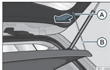
Fig. 109 Nel bagagliaio: smontare e montare il ripiano.
