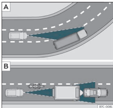
Fig. 159 A Veicolo in curva. B Motociclista che circola anteriormente fuori dal raggio d'azione del sensore radar.
