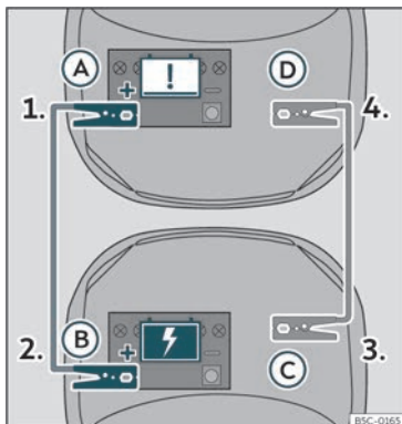
Fig. 42 Schema elettrico per i veicoli con sistema Start/Stop.
